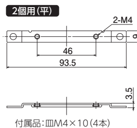
付属品: 皿M4×10 (4本)
