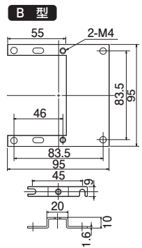
付属品: なべM4×5 (2本) なべM4×8 (4本)
