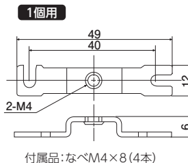
付属品: なべM4×8 (4本)
