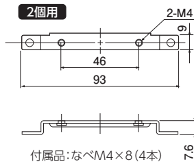
付属品: なべM4×8 (4本)
