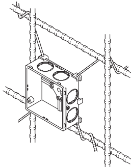
バーを曲げての取付け
