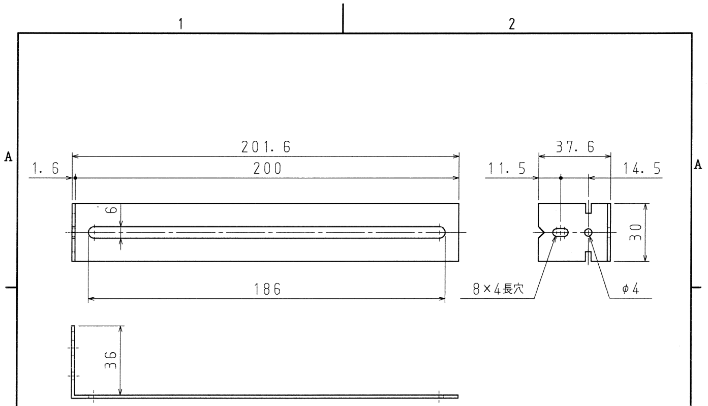
固定金具
